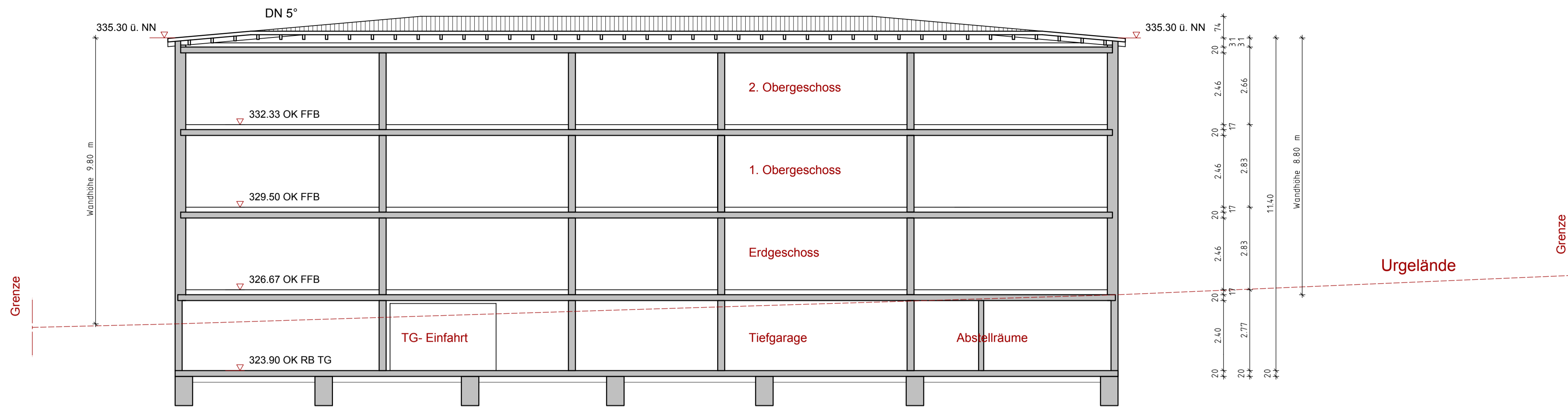
Schnitt A - A
