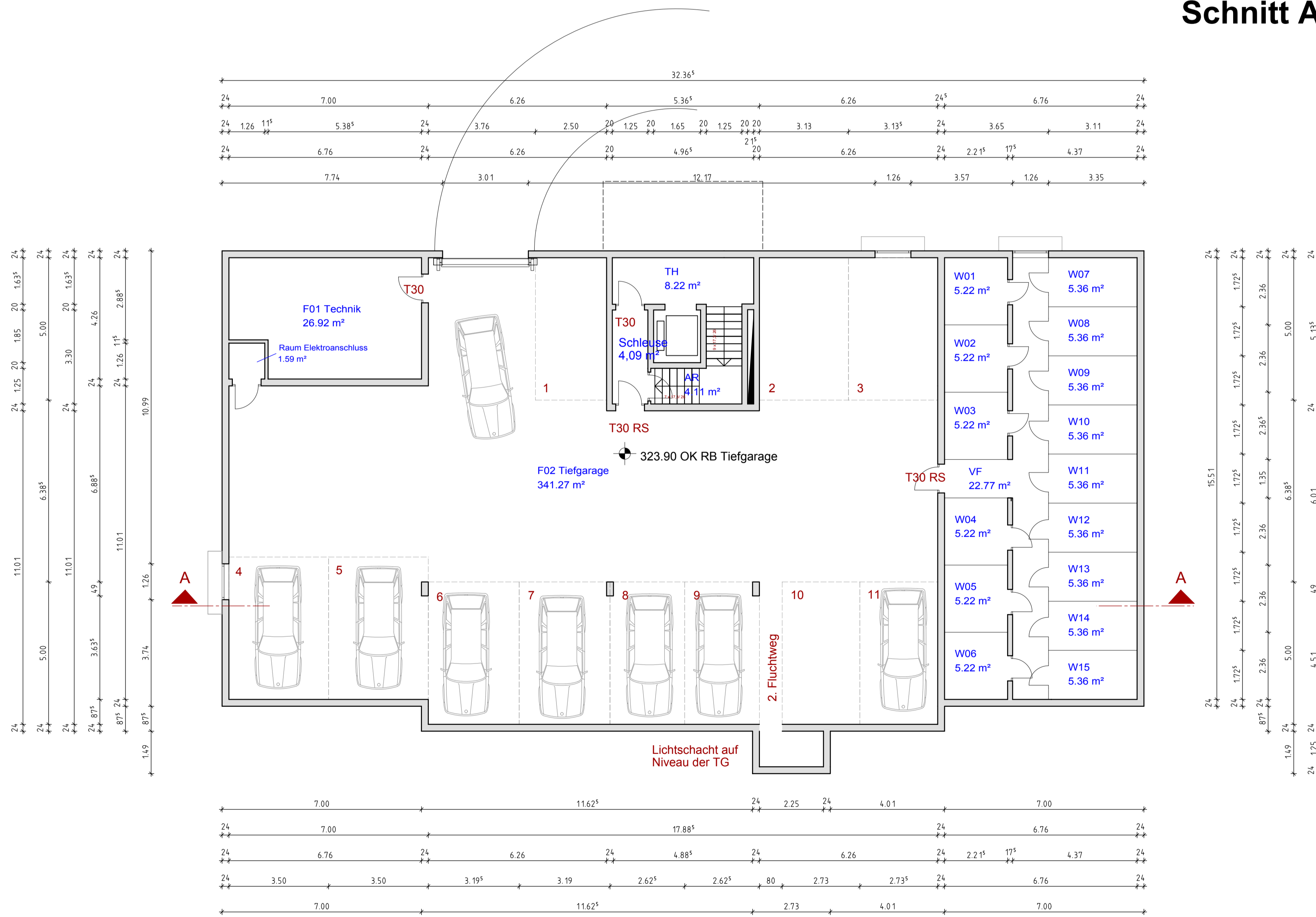
Grundriss Kellergeschoss
